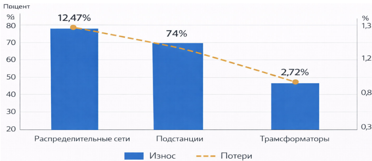
Рисунок 2. Уровень износа и технологических потерь в электросетевой инфраструктуре Республики Узбекистан
